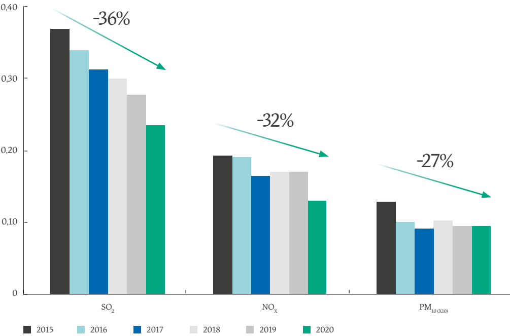
Δείκτες για τις Εκπομπές Διοξειδίου του Θείου (SO 2 ), Οξειδίων του Αζώτου (NO x ) και Σωματιδίων (PM 10 ) (kg εκπομπών ανά τη τροφοδοσίας από 2015 έως 2020)
