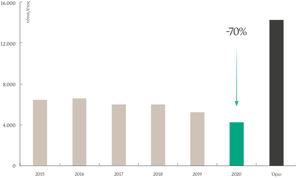
Σύγκριση εκπομπών Διοξειδίου του Θείου (SO 2 ) 2015-2020 με το ισχύον όριο
